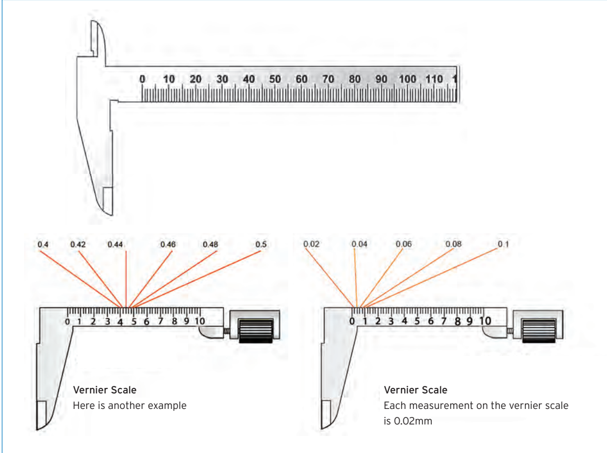
تقسيمات الورنية
