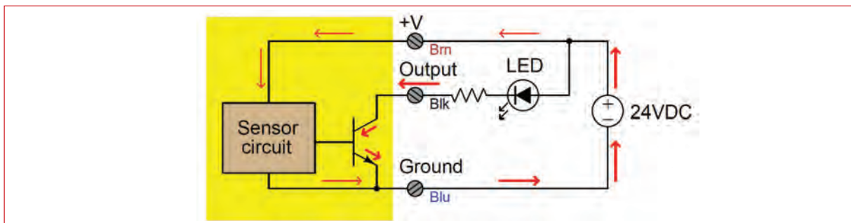
الرسومات الكهربائية
